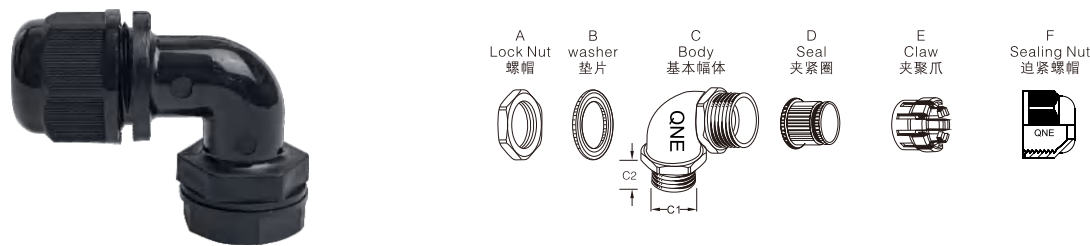
E-27 90°尼龙电缆防水接头（分体）
