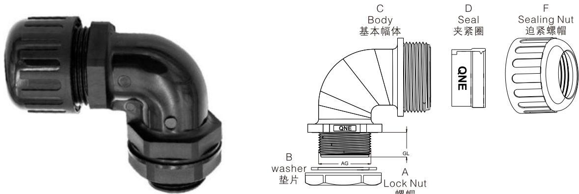
E-26 90°C防水浪管接头
